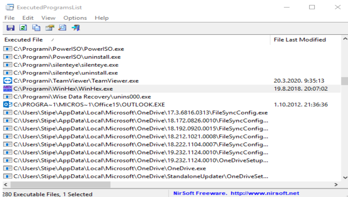
Slika 22. ExecutedProgramsList
