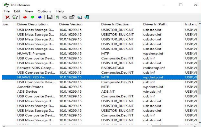
Slika 17. USBDeview
