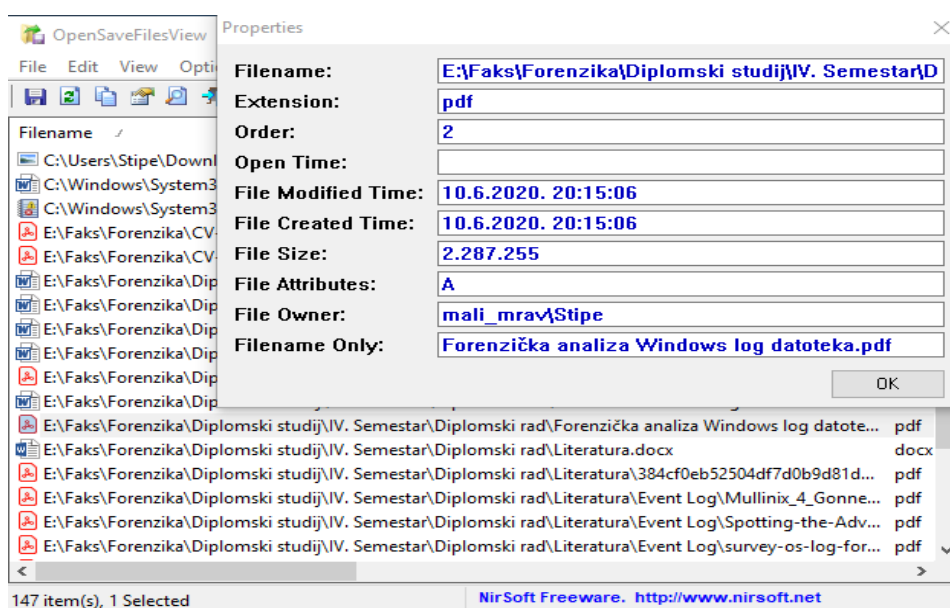
Slika 23. OpenSaveFilesView
