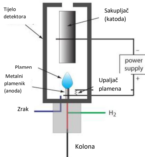
Slika 15. Plameno-ionizacijski detektor
