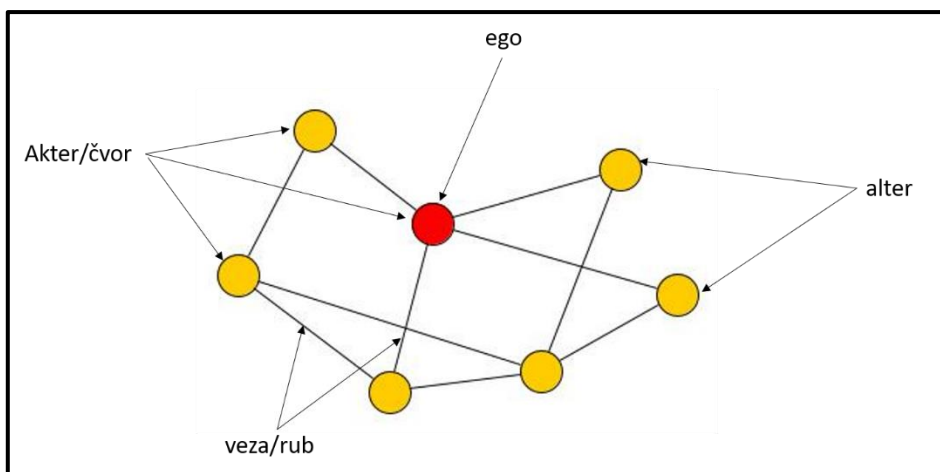
Slika 3 Primjer ego-mreže
